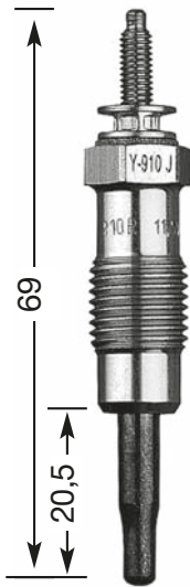
Y-910 J M 12 x 1.25 12 Hex 11,5 V DP 3
