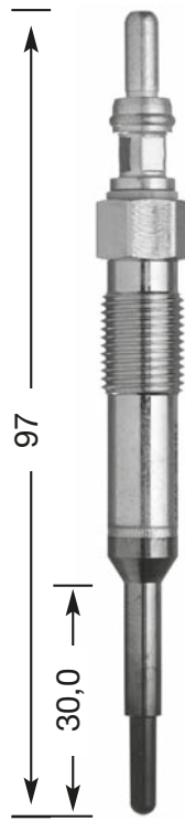
CZ 104 M 10 x 1.0 10 Hex 7 V
