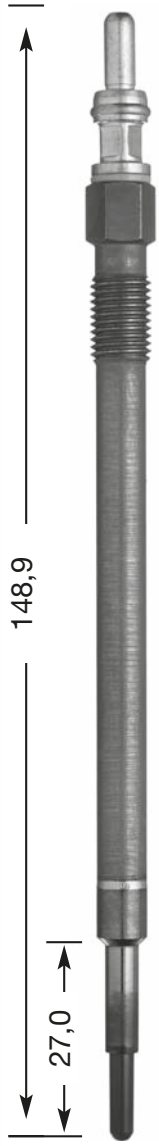
CZ 303 M 8 x 1.0 8 Hex 7 V DP 54
