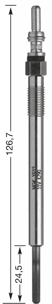
YE 12 M 8 x 1.0 8 Hex 11 V
