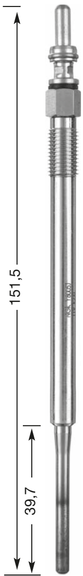
Y8005 J M 8 x 1.0 8 Hex 11 V DP 64
