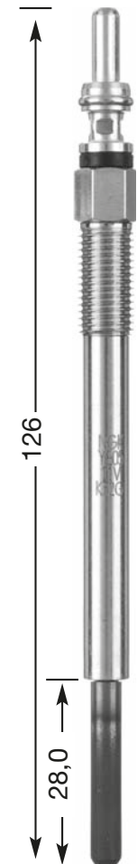
YE 05 M 8 x 1.0 8 Hex 11 V DP 73
