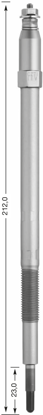
CZ 258 M 10 x 1.25 12 Hex 11 V
