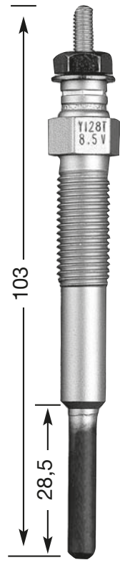
Y-128 T M 10 x 1.25 12 Hex 8,5 V
